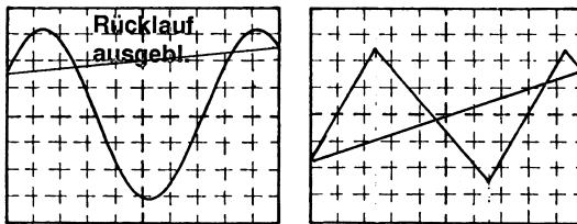
Abb. 2.8: Rückstrahl Ausblendung (Dunkelsteuerung)
