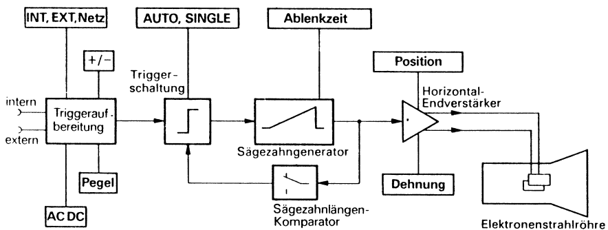
Abb. 2.11: Blockschaema des horizontalen Ablenk- und Verstärkersystems
