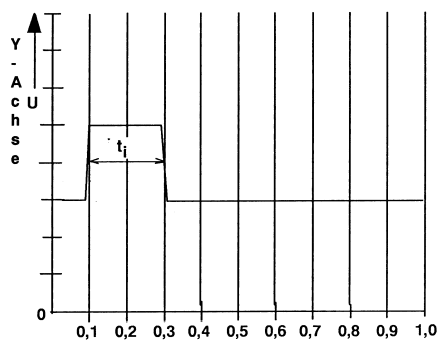
c) 0,1 ms/DIV X-Achse t →
