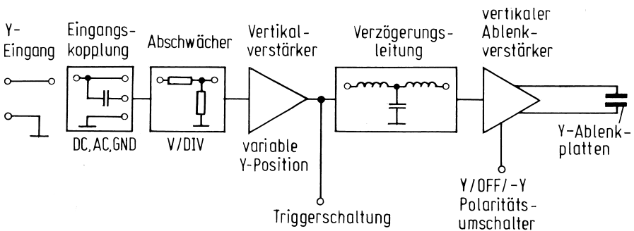
Abb. 2.9: Blockschaubild des Vertikalverstärkersystems
