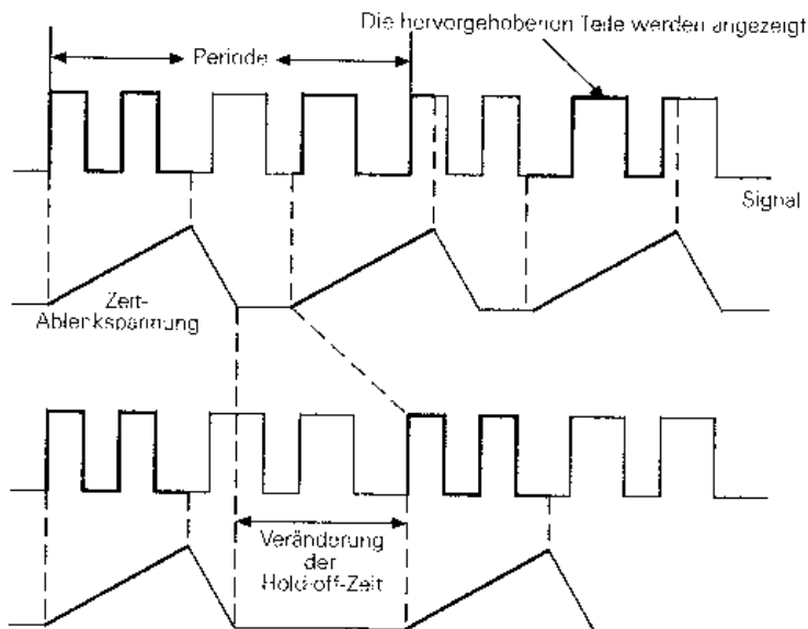
Abb. 2.18: Hold-off-Funktion
