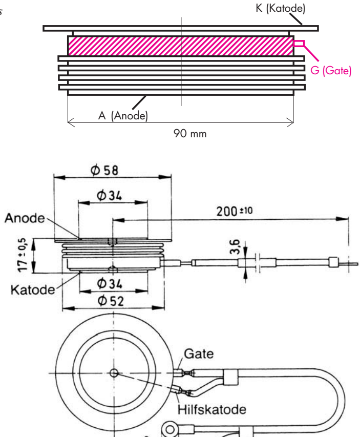
Bild 2.8b Gehäuse eines Thyristors mit Anschlüssen (Scheibengehäuse)
