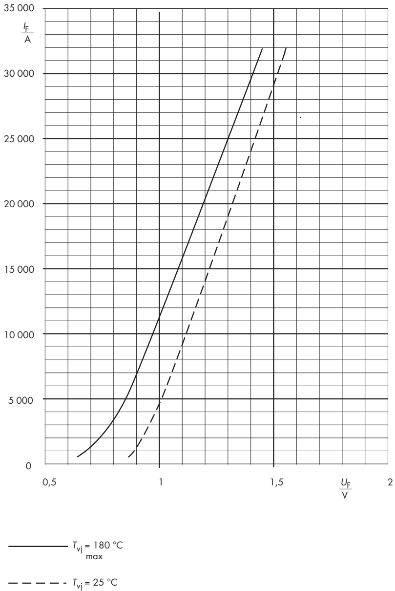
Bild 2.3b Durchlasskennlinie einer Leistungsdiode
