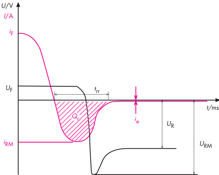
Bild 2.4 Ausschalten einer Leistungsdiode
