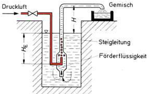
Bild 1.7 Arbeitsprinzip einer Mammutpumpe
