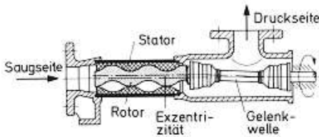
Bild 1.6 Exzentrerschneckenpumpe
