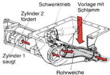
Bild 1.5 Dickstoff-Rohrweichen-Kolbenpumpe (nach Putzmeister)
